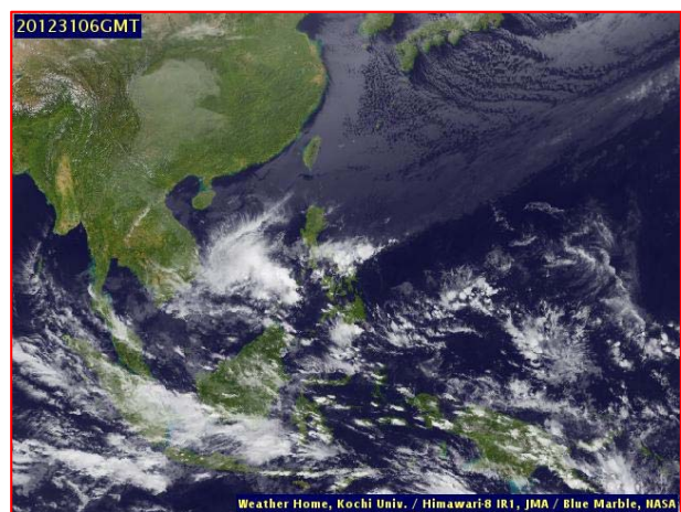
ภาพถ่ายดาวเทียม วันที่ ๓๑ ธ.ค. ๒๕๖๓ เวลา ๑๓.๐๐ น.
